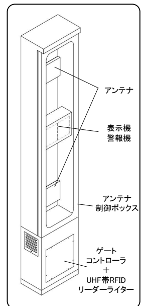
アンテナ制御ボックス タイプ概観
